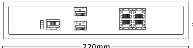
220mm 前视图
